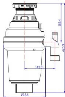
WDU 800 AIR
